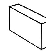
КЕРАМЗИТОБЕТОННЫЙ 390 x 90 x 188 мм
